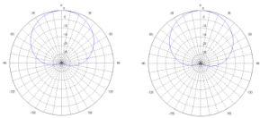
水平面方向图 Horizontal pattern
