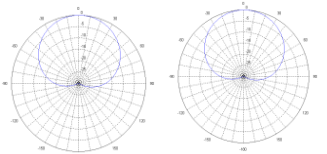
水平面方向图 Horizontal pattern
