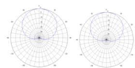
水平面方向图 Horizontal pattern
