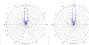
垂直面方向图 Vertical pattern
