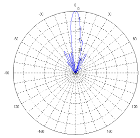
垂直面方向图 Vertical pattern
