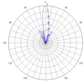
垂直面方向图 Vertical pattern
